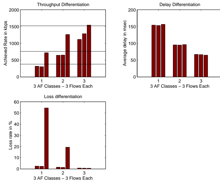
Figure 14. Original HPD: CBR/UDP and Pareto/TCP
